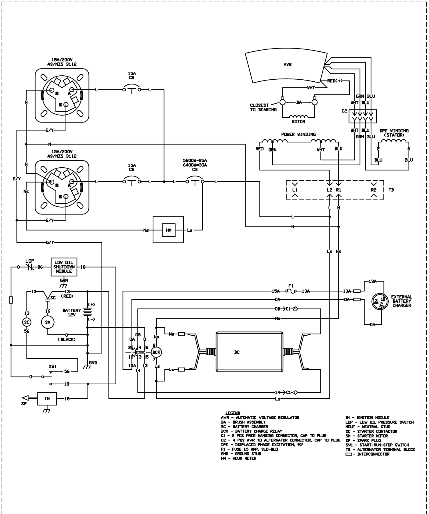
SCHEMATIC - DIAGRAM WD SD XP5600E/6400E 50HZ AUS DRAWING #: 0K2042
