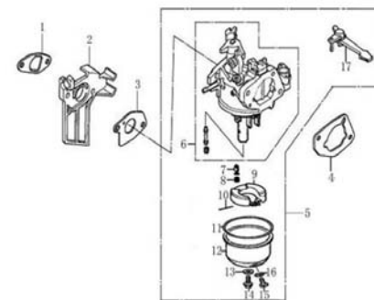
化油器(CARBURETOR)
