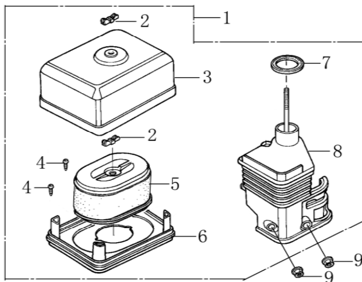
空滤器 ( AIR CLEANER )
