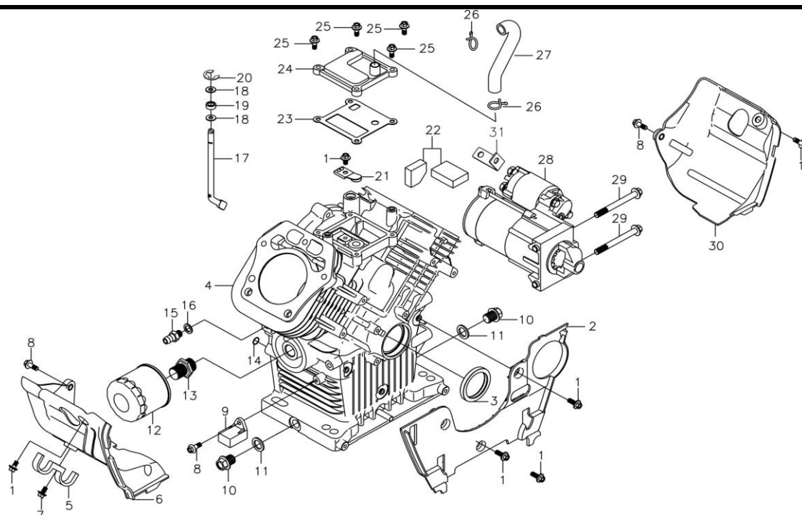
曲轴箱体（CRANKCASE）
