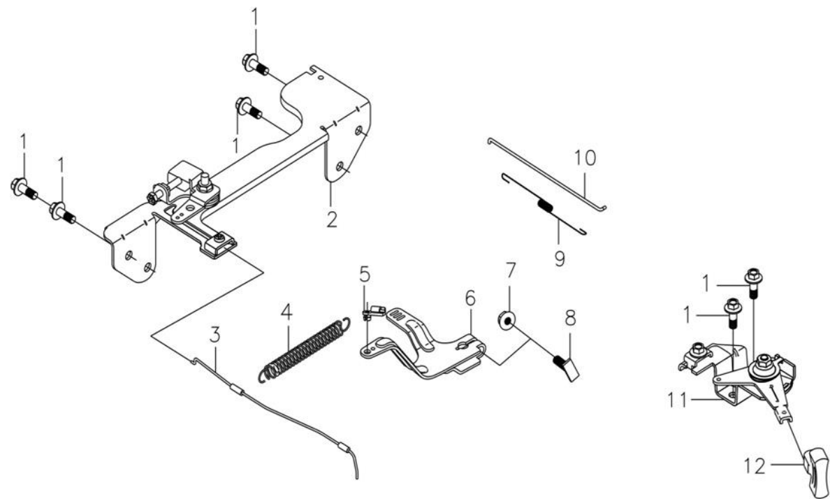
调速控制（CONTROL）
