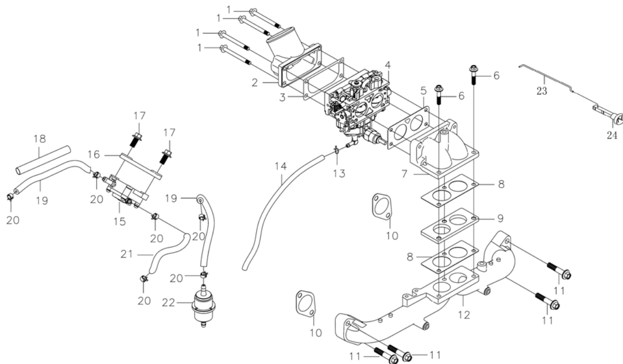
化油器 (CARBURETOR)
