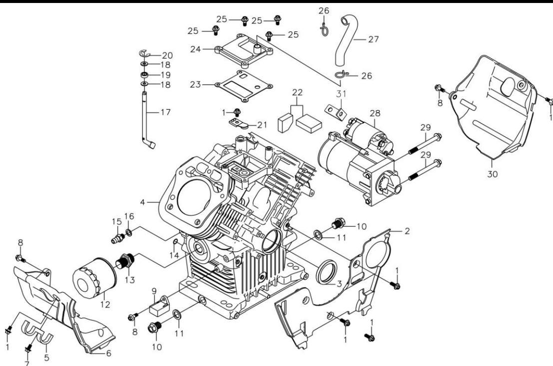
曲轴箱体（CRANKCASE）
