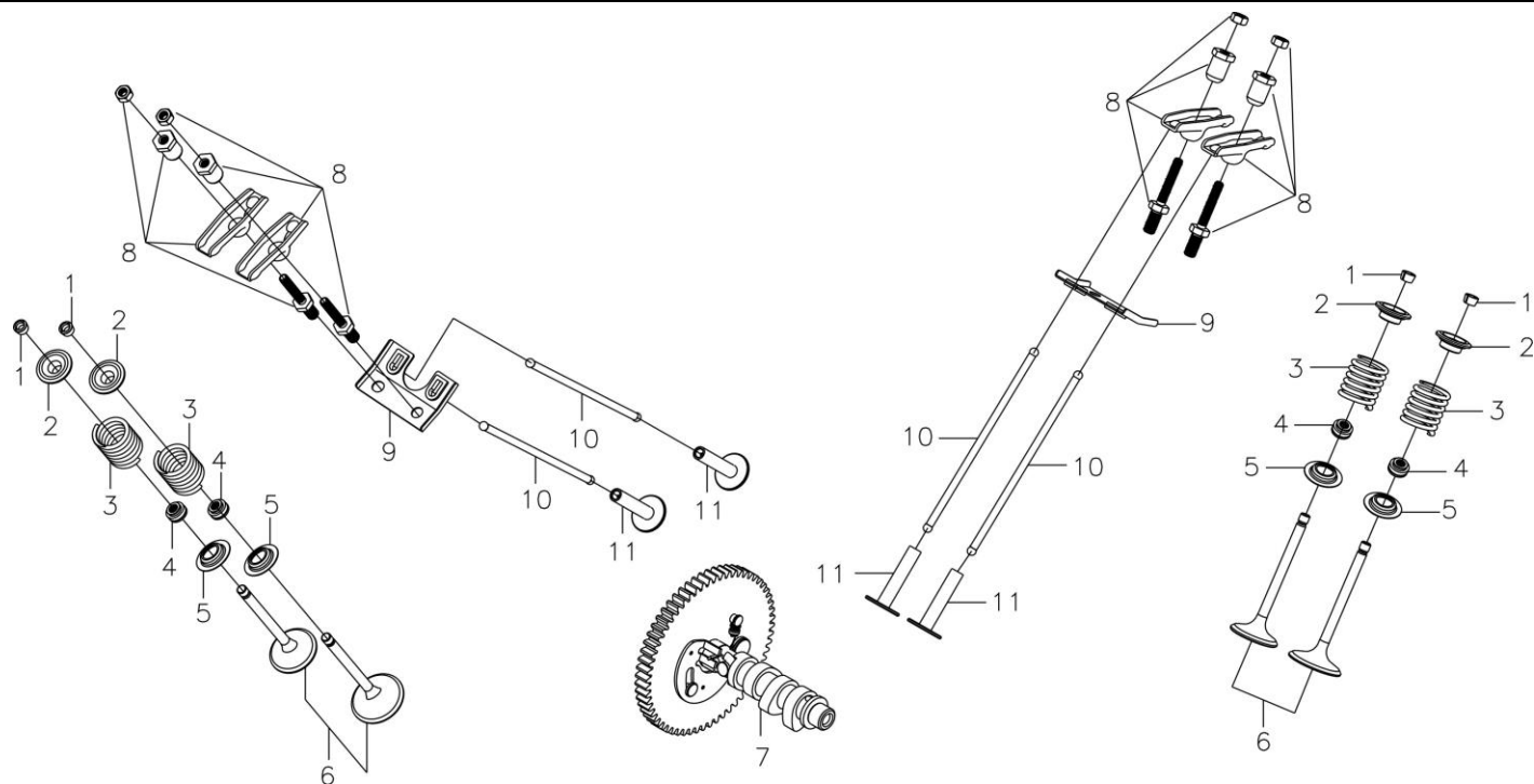
配气系统 (ROCKER,CAMSHAFT)
