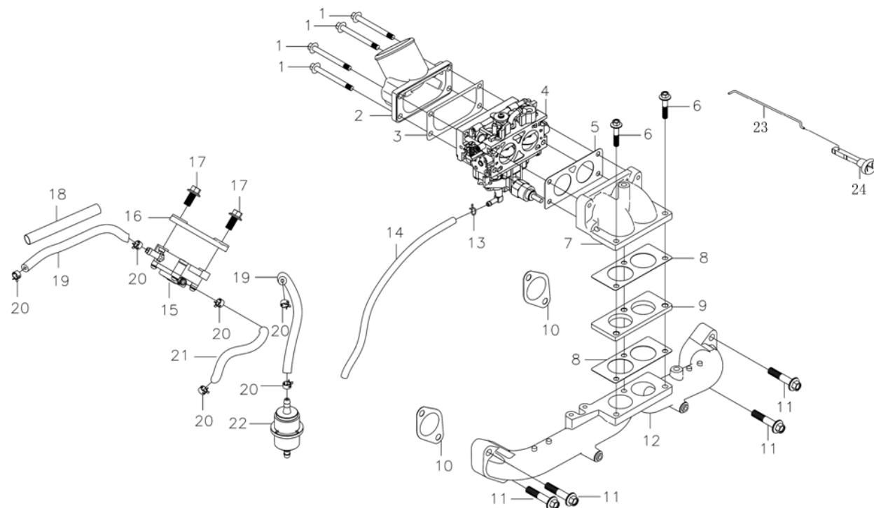
化油器 (CARBURETOR)
