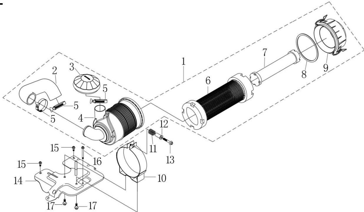
空滤器（AIR CLEANER）
