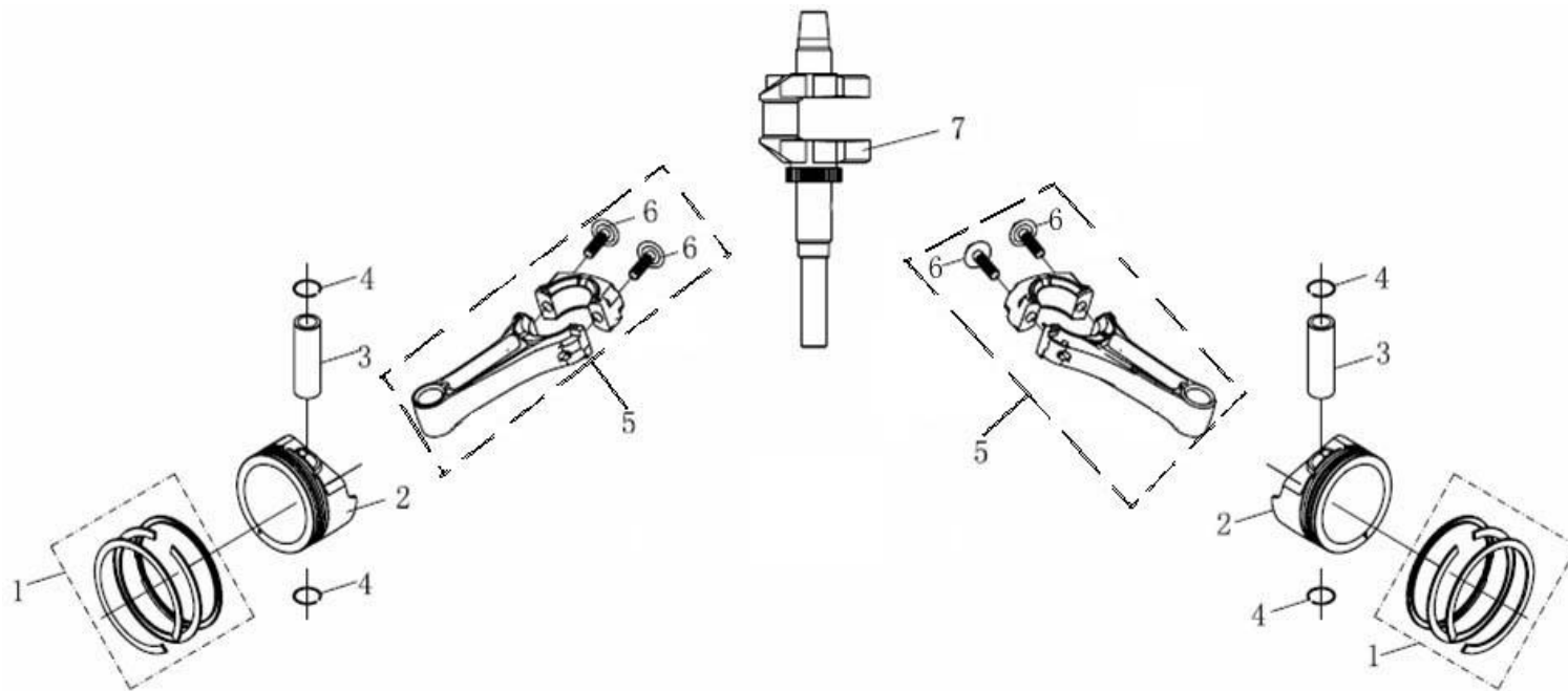
曲轴活塞组件 (Crankshaft/Piston)
