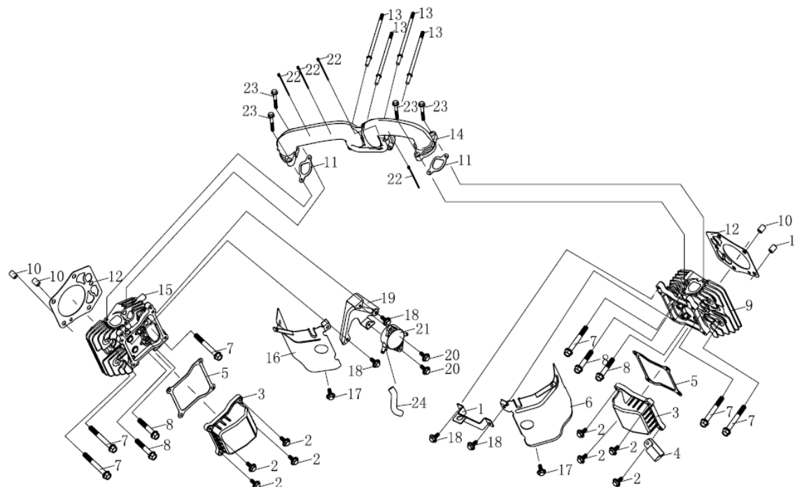
气缸头组件 (Cylinder Head)
