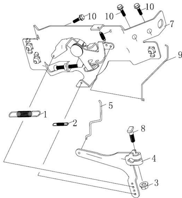
调速控制系统 (Governor)
