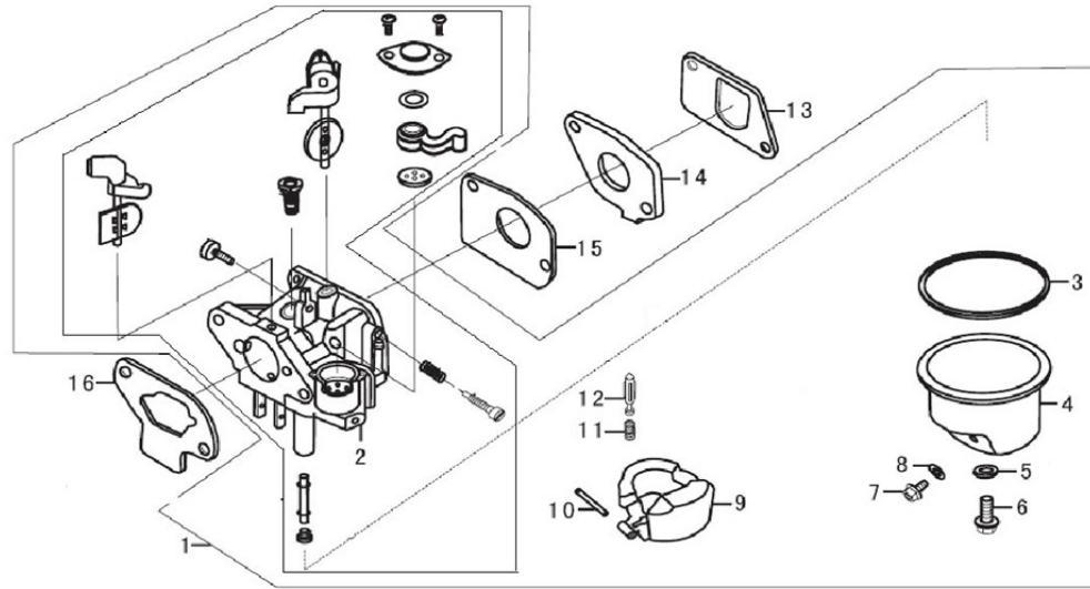
化油器 CARBURETOR
