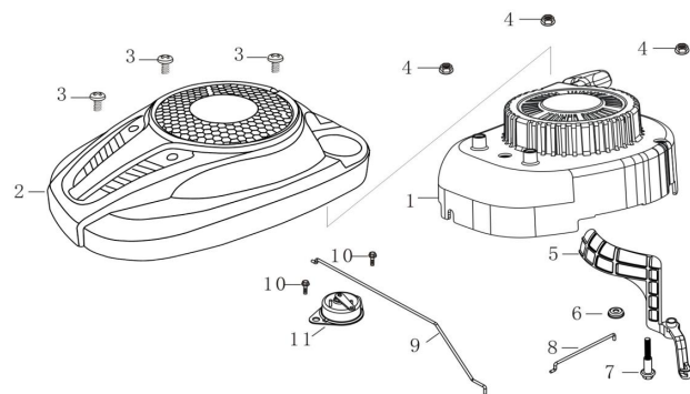
起动器 (Starter) Auto Choke Version
