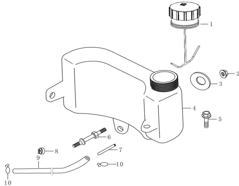
油箱 (FUEL TANK)
