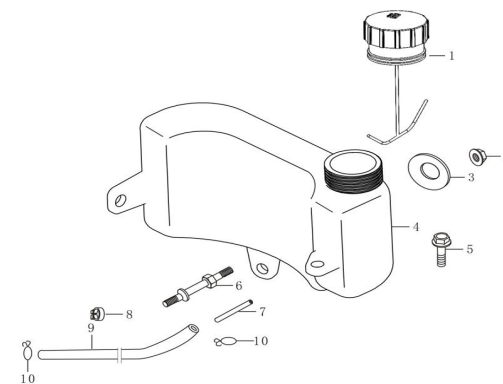
油箱 (Fuel Tank)
