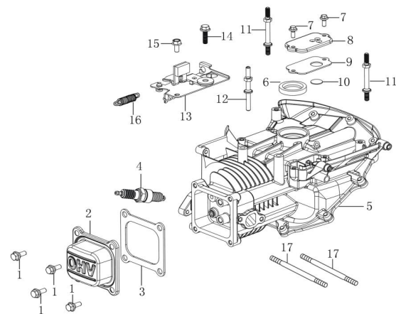
曲轴箱（Crankcase）
