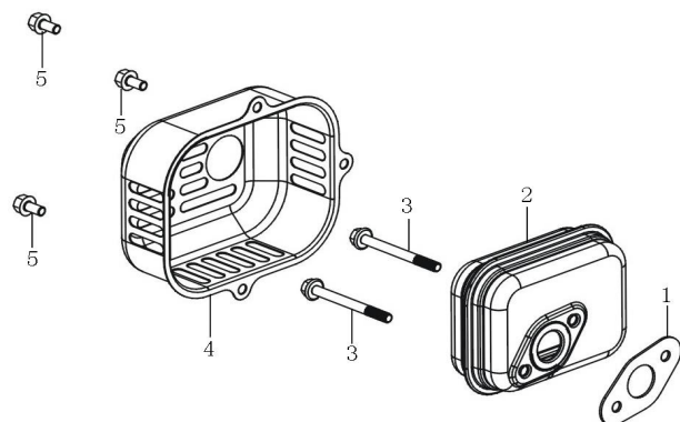
消声器 (Muffler)
