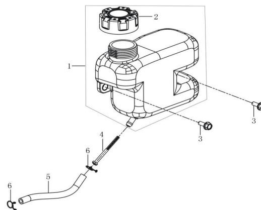
油箱 (Fuel Tank)
