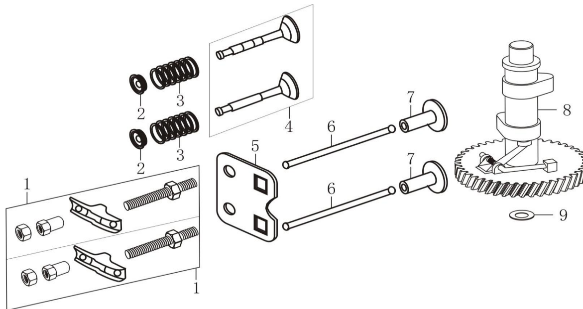
配气机构 (CAMSHAFT)
